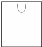
Vertical Tasche Format: 400x160x450 mm Anzahl pro Karton: 50 St. Menge auf der Palette: 1800 St.
