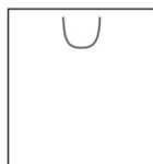
torba pionowa format: 400x250x450 mm ilość w kartonie: 50 szt. ilość na palecie: 800 szt.
